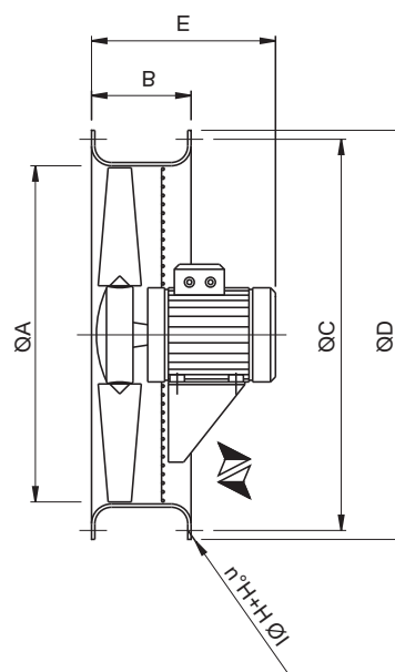
RING drp-g
