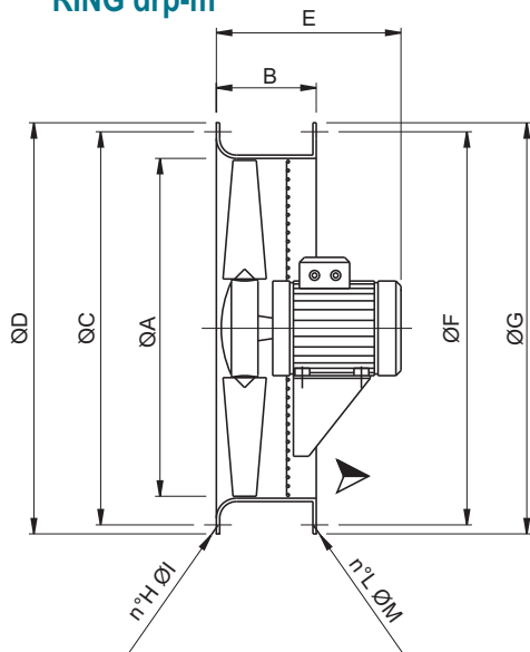
RING drp-m
