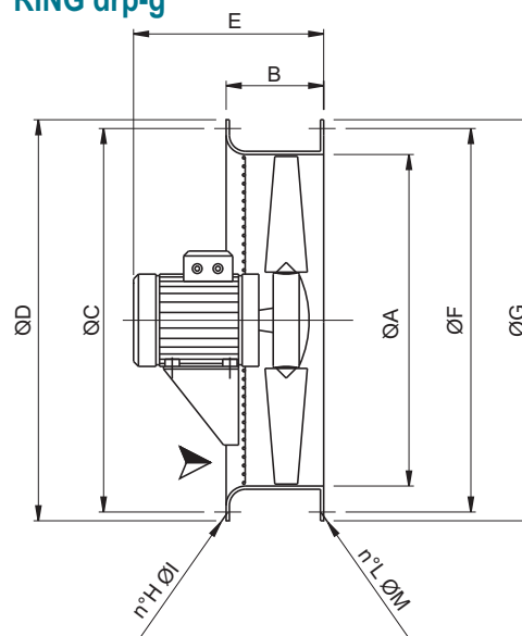
RING drp-g
