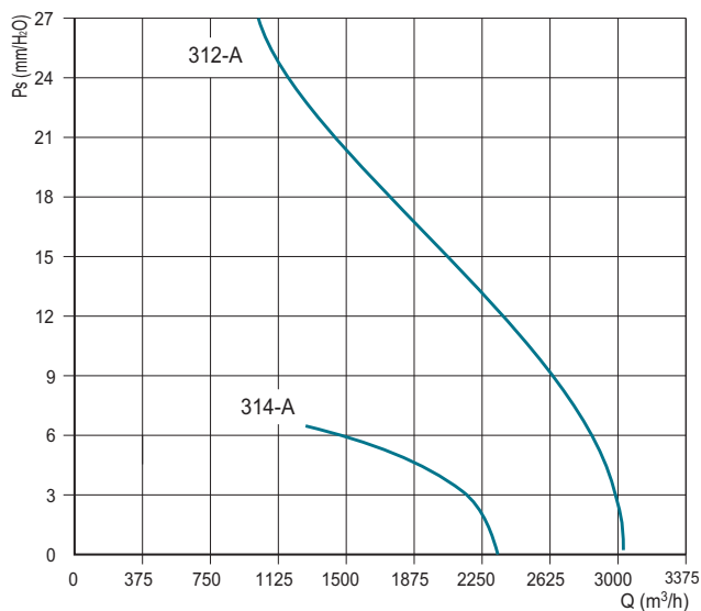
DUCT-M 310
