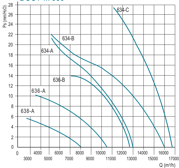
DUCT-M 800 - 4 poles
